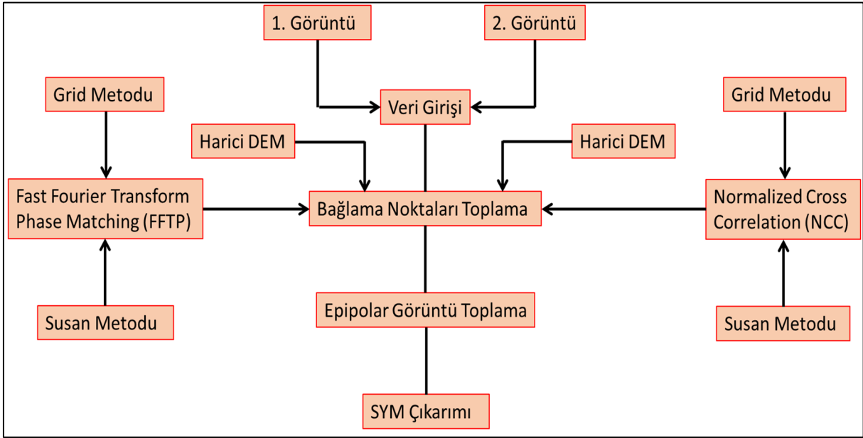
Şekil 4. Stereo Görüntülerden SYM Üretimi İş Adımları.
